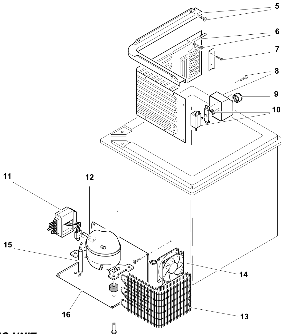
BI 40 - COOLING UNIT
